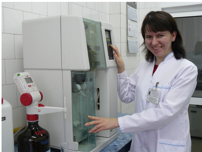
Na zdjęciu: analiza próbek nawozów naturalnych – destylacja azotu.
